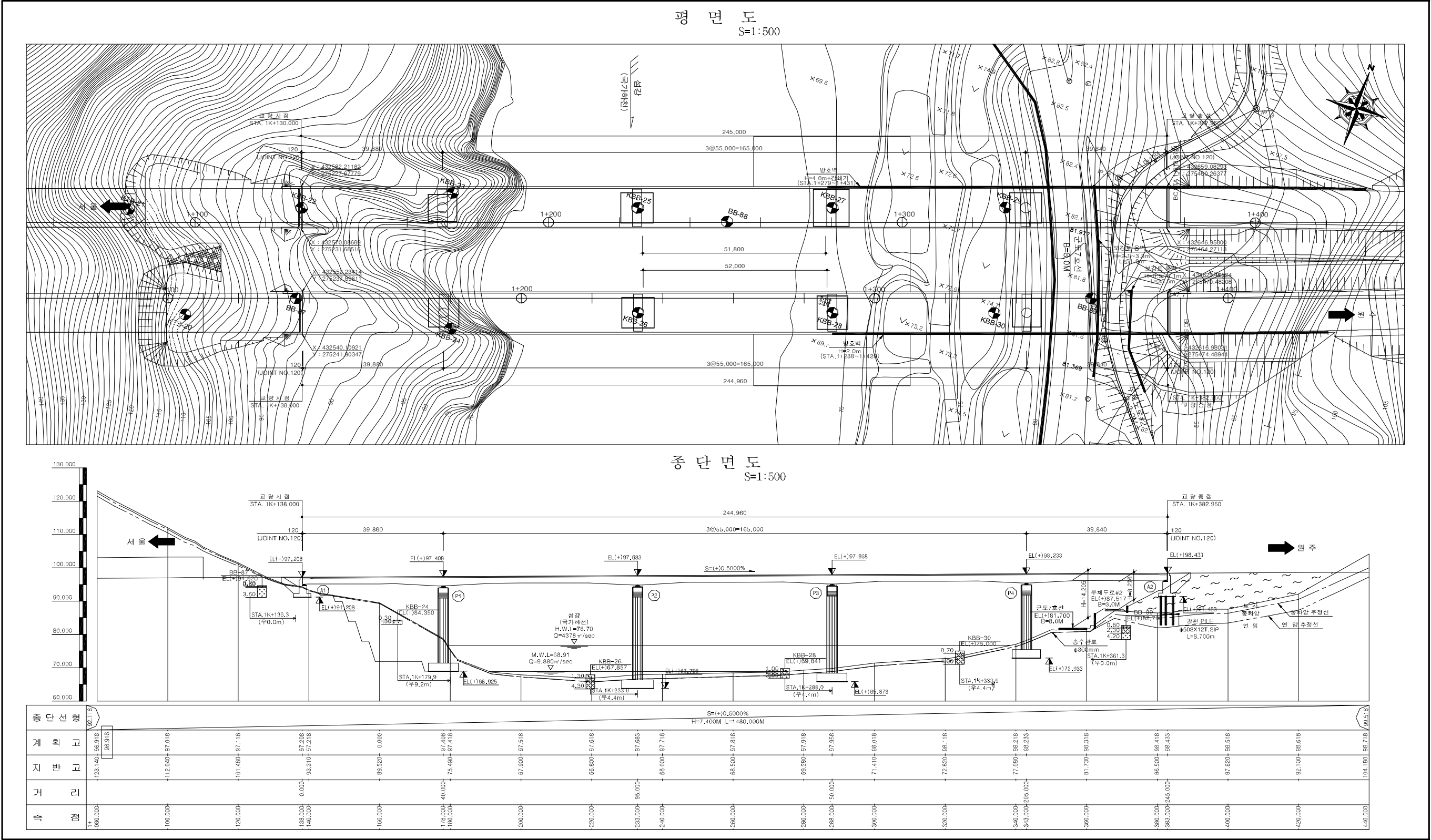
【그림 1.3-1】 중평면도
