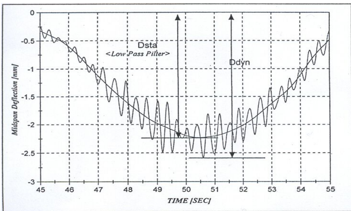
【그림 4.2-10】 처짐이력곡선
