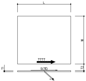
슬플레이트 상세 S=1:30
