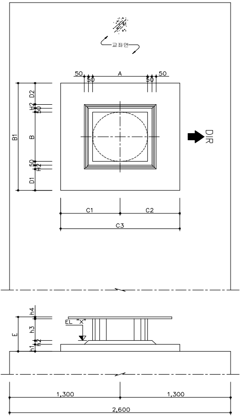
슬플레이트 상세 S=1:30
